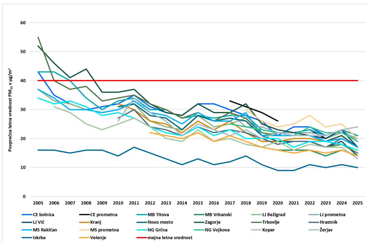
Slika 3: Povprečne letne ravni delcev PM 10 v zraku v obdobju od leta 2005 do 2025 na posameznih merilnih mestih DMKZ v Sloveniji (Vir podatkov: ARSO).
