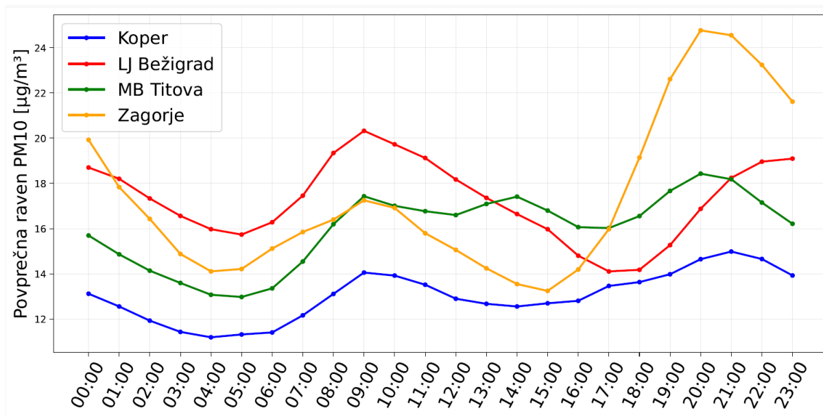
Slika 1: Dnevni potek povprečne urne ravni PM 10 na izbranih merilnih mestih v kurilni sezoni leta 2025 (januar do marec in oktober do december). (Vir podatkov: ARSO.)
