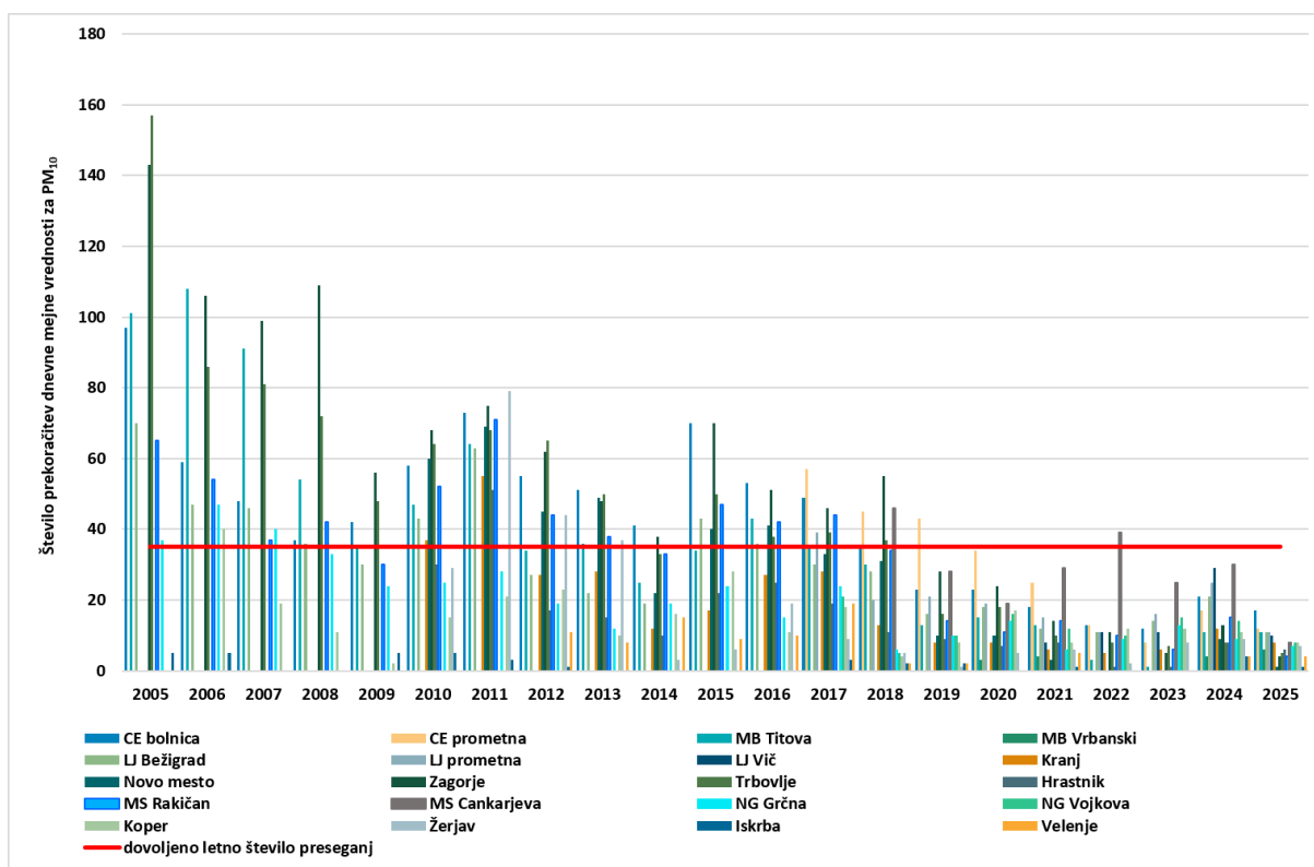
Slika 2: Število prekoračitev dnevne mejne vrednosti delcev PM 10 v zraku v obdobju od leta 2005 do 2025 na posameznih merilnih mestih DMKZ v Sloveniji (Vir podatkov: ARSO).
