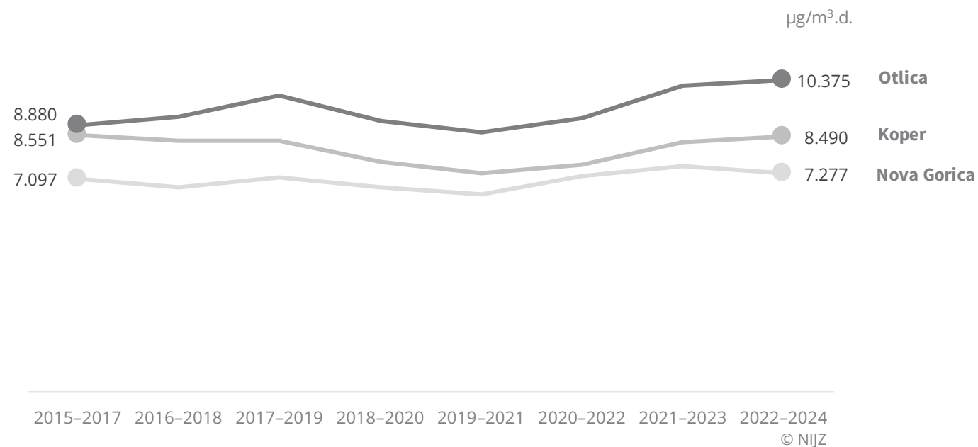
3.6.2.Slika 5: Drseče triletno povprečje kazalca SOMO_{35} na merilnih mestih Otlica, Koper in Nova Gorica, 2015–2024
