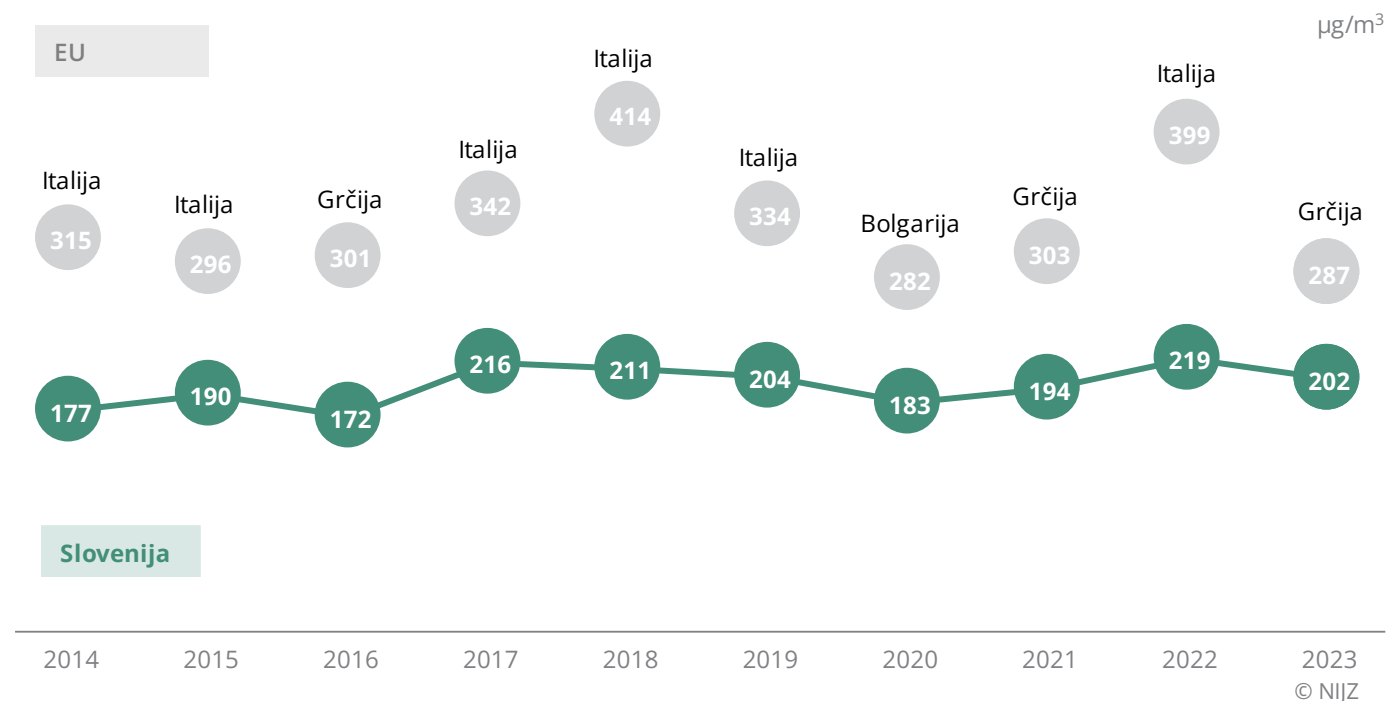
3.6.2.Slika 6: Maksimalne urne ravni ozona , Slovenija in EU, 2014–2023
