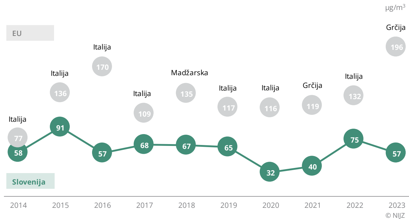
3.6.2.Slika 7: Število dni s preseženo ciljno vrednostjo za ozon, Slovenija in EU, 2014–2023
