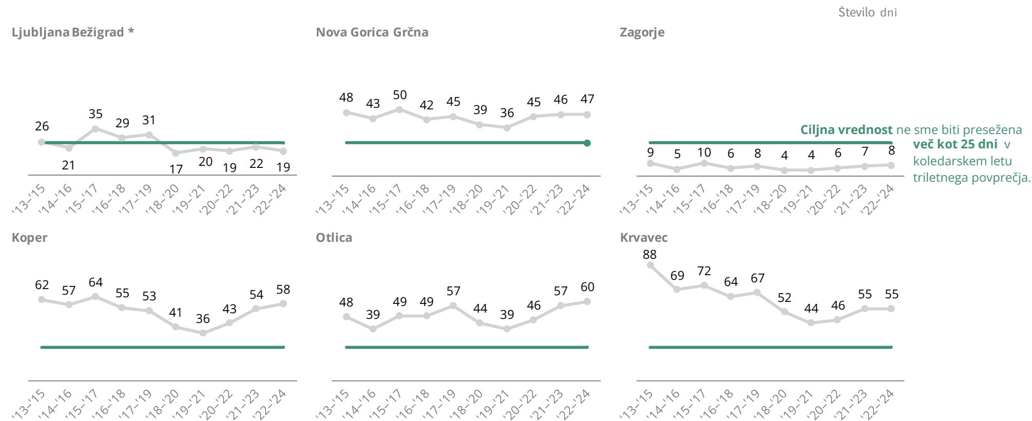
3.6.2.Slika 4: Število dni s preseženo ciljno vrednostjo za ozon v triletnem povprečju, na merilnih mestih DMKZ, triletna obdobja od 2013–2015 do 2022–2024
