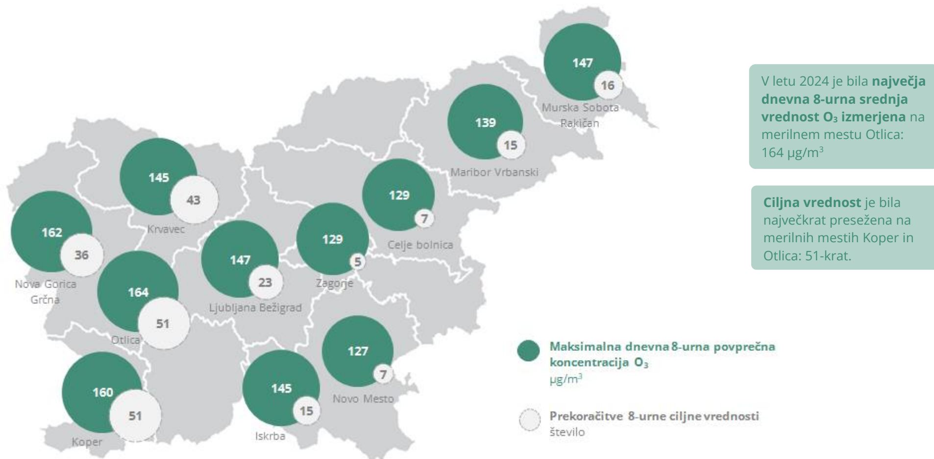
3.6.2.Slika 1: Največja dnevna 8-urna srednja vrednost O_3 in število prekoračitev ciljne vrednosti po merilnih mestih DMKZ, Slovenija, 2024
