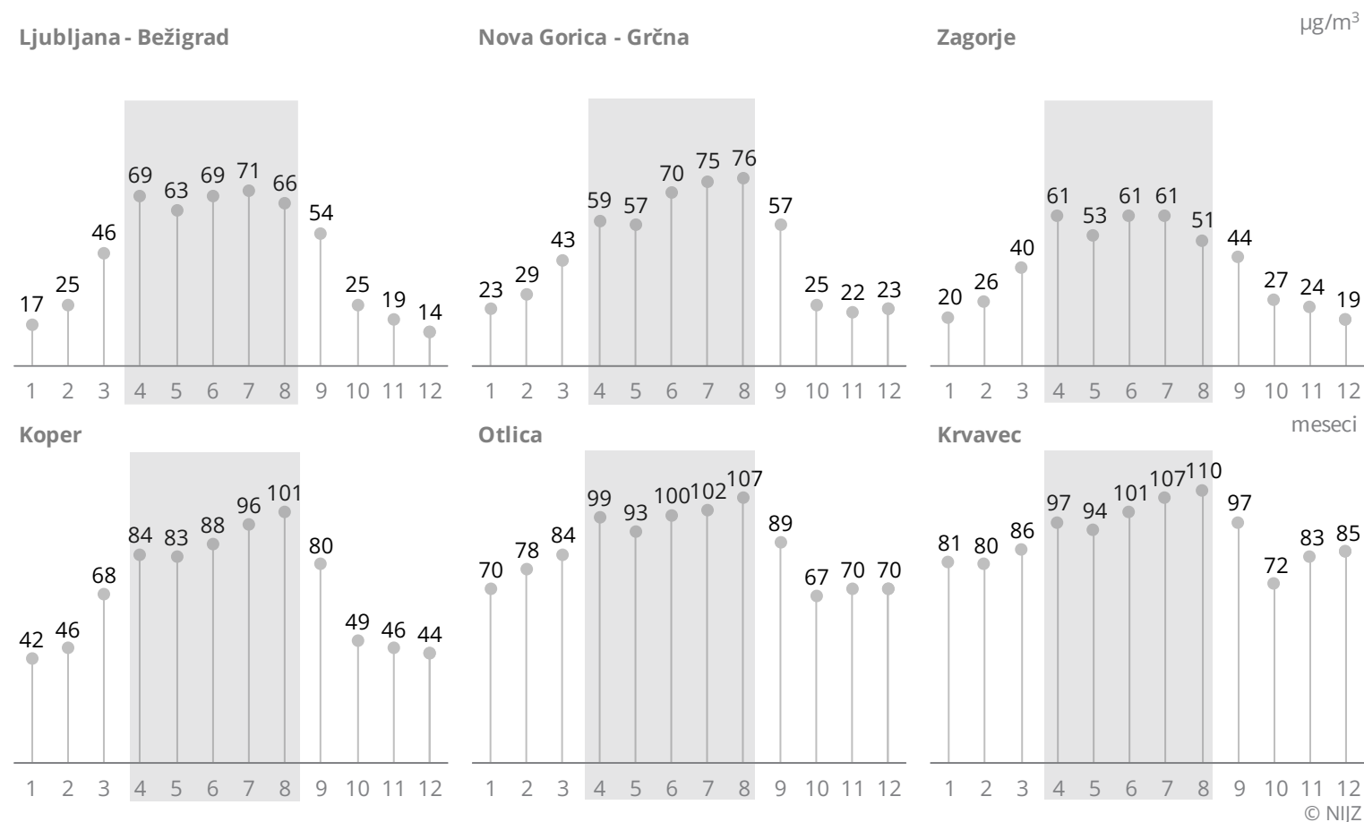
3.6.2.Slika 3: Letni hod ozona na nekaterih merilnih mestih DMKZ, Slovenija, 2024
