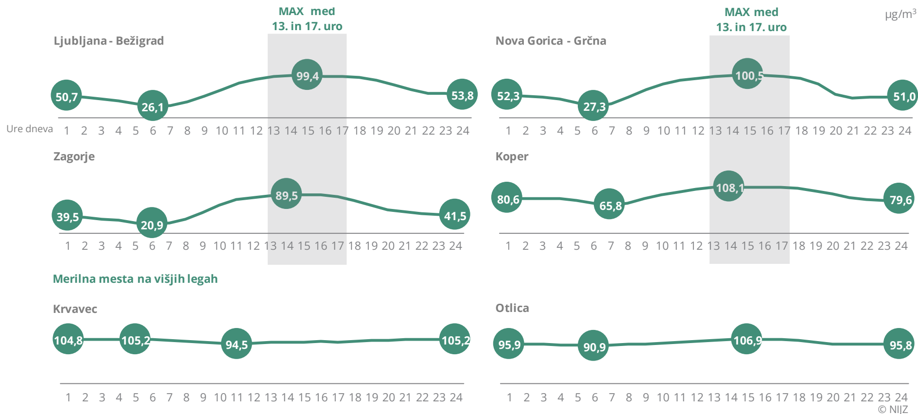
3.6.2.Slika 2: Dnevni hod ozona na nekaterih merilnih mestih DMKZ, Slovenija, april - september 2024
