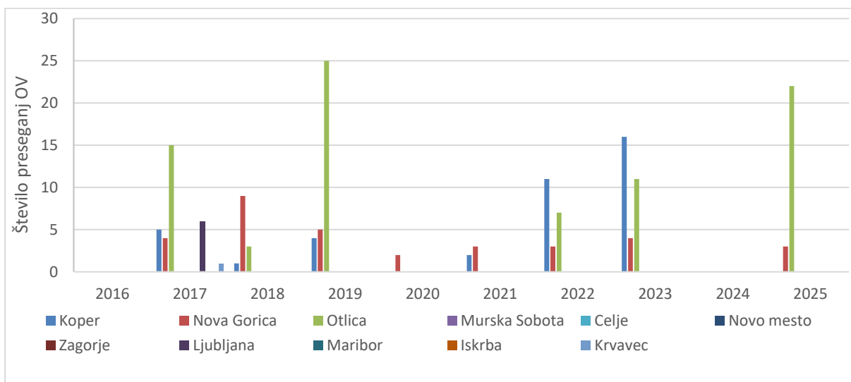
Slika 2. Število preseganj opozorilne vrednosti (OV) za ozon v različnih slovenskih krajih v obdobju od leta 2016 do 2025. Opozorilna vrednost znaša 180 \mu\text{g}/\text{m}^3 in je postavljena z namenom zaščititi prebivalstvo pred kratkotrajno izpostavljenostjo visokim koncentracijam ozona (vir podatkov: ARSO, 2026)
