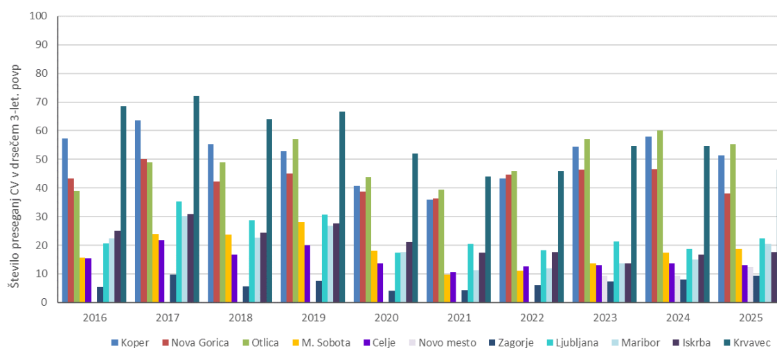
Slika 1. Število preseganj ciljne vrednosti (CV) za ozon v različnih slovenskih krajih v drsečem povprečju treh let za obdobje 2016–2025 (leto 2016 predstavlja prvo triletno obdobje 2014-2016). Ciljna vrednost znaša 120 µg/m 3 in ne sme biti presežena več kot 25 dni v koledarskem letu, računano v drsečem povprečju treh let (vir podatkov: ARSO, 2026)
