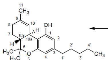
\Delta^9 -THC
