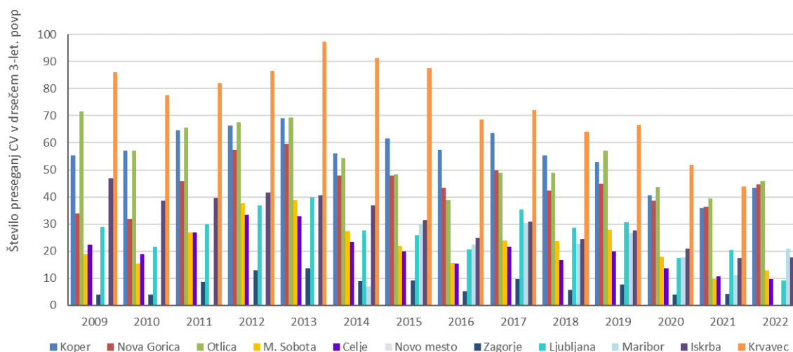
Slika 1. Število preseganj ciljne vrednosti (CV) za ozon v različnih slovenskih krajih v drsečem povprečju treh let za obdobje 2007–2022 (leto 2009 predstavlja prvo triletno obdobje 2007-2009). Ciljna vrednost znaša 120 \mu\text{g}/\text{m}^3 in ne sme biti presežena več kot 25 dni v koledarskem letu, računano v drsečem povprečju treh let (vir podatkov: ARSO, 2023)
