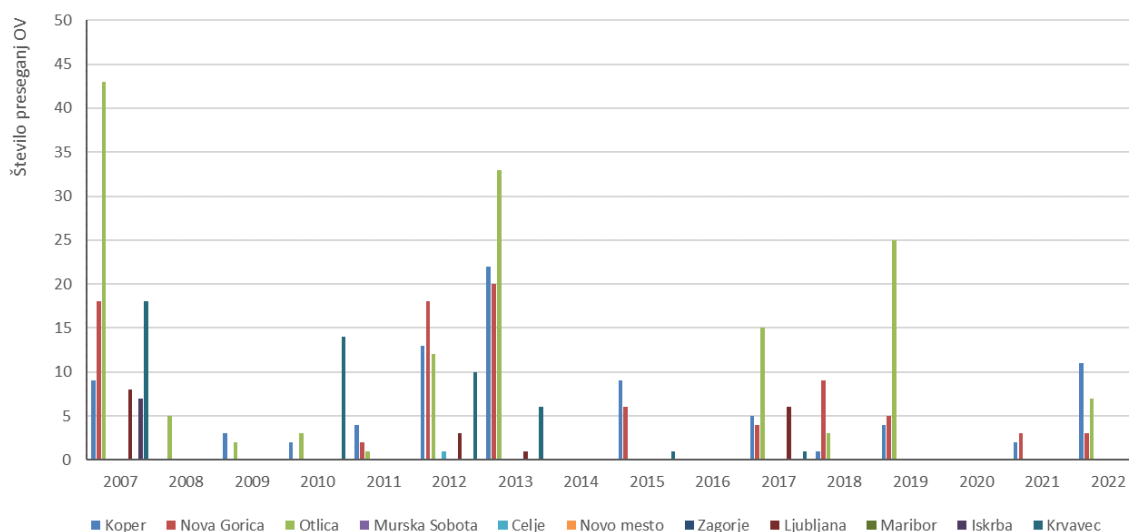
Slika 2. Število preseganj opozorilne vrednosti (OV) za ozon v različnih slovenskih krajih v obdobju od leta 2007 do 2022. Opozorilna vrednost znaša 180 \mu\text{g}/\text{m}^3 in je postavljena z namenom zaščiti prebivalstvo pred kratkotrajno izpostavljenostjo visokim koncentracijam ozona (vir podatkov: ARSO, 2023)
