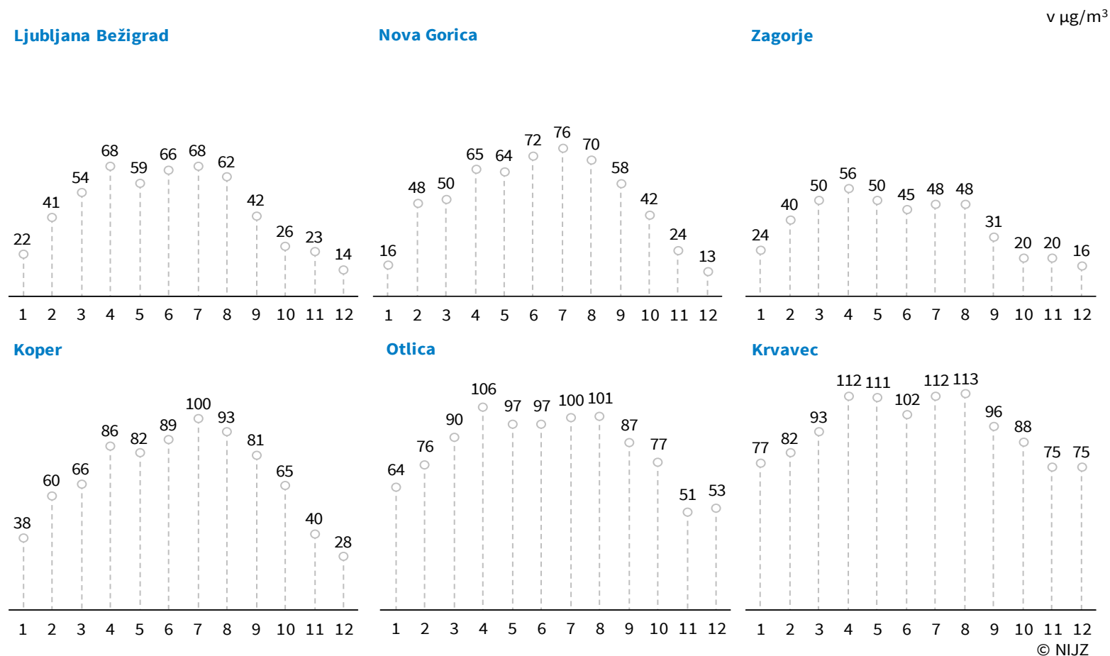
3.7.2 Slika 2: Letni hod ozona na nekaterih merilnih mestih DMKZ, Slovenija, 2018
