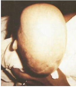
Slika 7.3: Skafocelija ali dolihocelija
