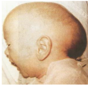
Slika 7.3: Skafocelija ali dolihocelija
