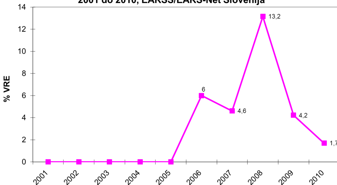
Pojavljanje proti vankomicinu odpornih izolatov E. faecium , 2001 do 2010, EARSS/EARS-Net Slovenija
