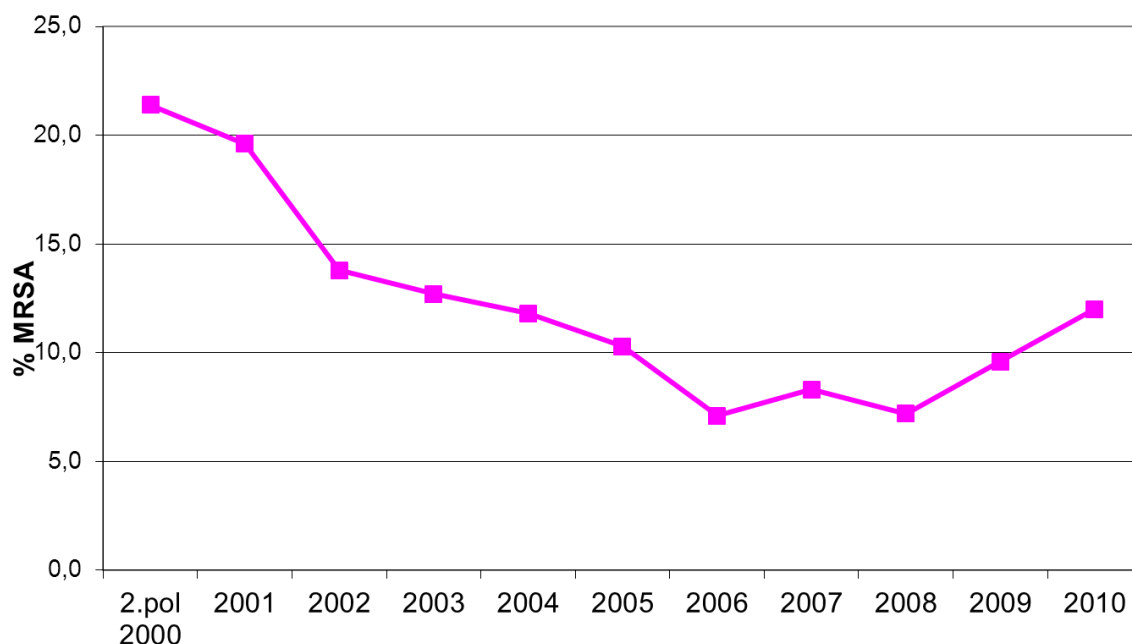
Odstotek MRSA izolatov med izolati S. aureus iz hemokultur, 2000 do 2010, EARSS/EARS-Net Slovenija
