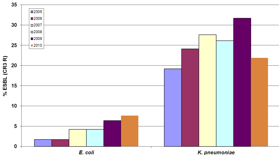
Odpornost proti cefalosporinom 3. generacije (CR3 R/ESBL) med izolati E. coli in K. pneumoniae , 2005 do 2010, EARSS/EARS-Net Slovenija
